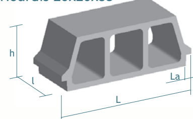
Hourdis 20x20x53
