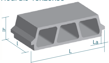
Hourdis 15x25x53
