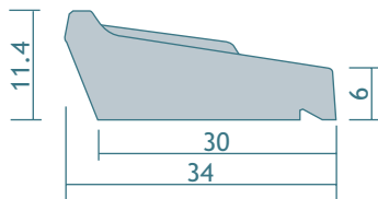
Appuis AL340
