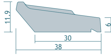
Appuis AL380
